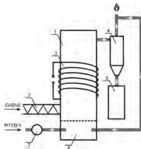
Рис. 1. Блок-схема опытной установки по термохимической переработке различных материалов методом пиролиза
