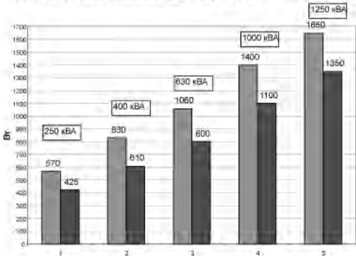
Сравнение потерь холостого хода трансформаторов ТМГ11 и ТМГ12
