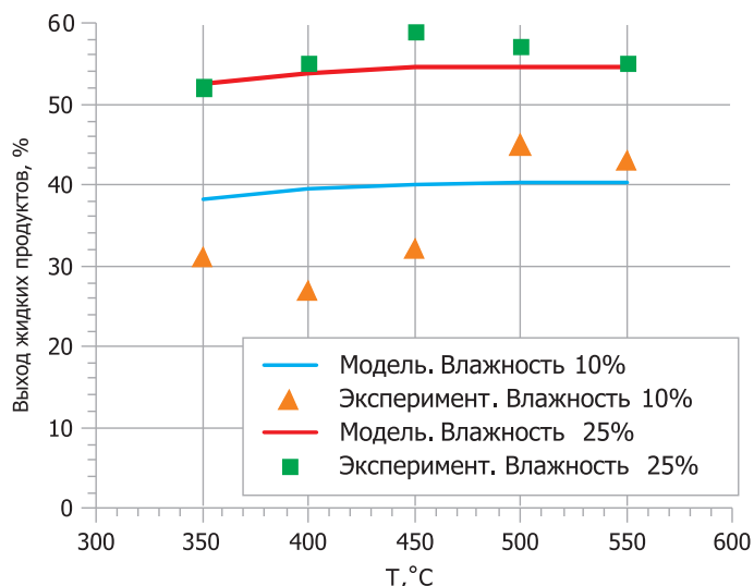
Рис. 3. Зависимость массового выхода жидких продуктов пиролиза от температуры кипящего слоя
