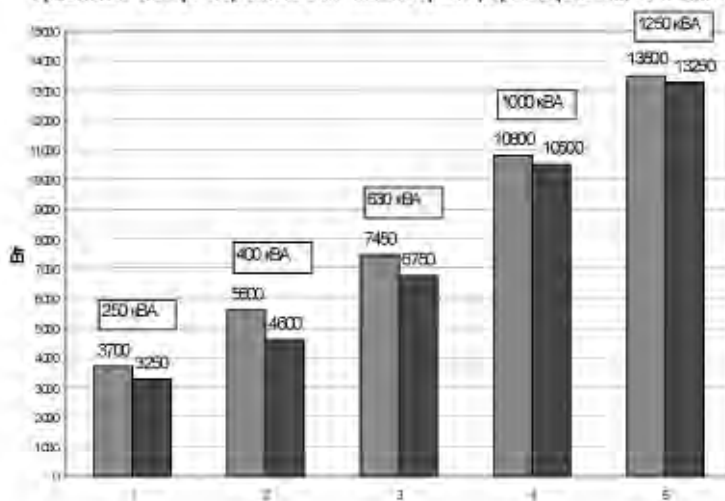
Сравнение потерь короткого замыкания трансформаторов ТМГ11 и ТМГ12
