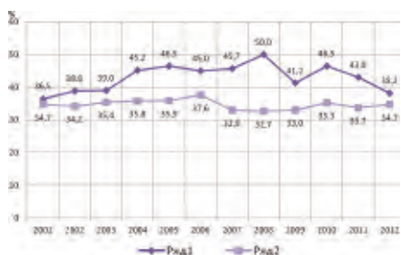
Рис 4. Динамика изменения коэффициентов использования установленной мощности турбин
