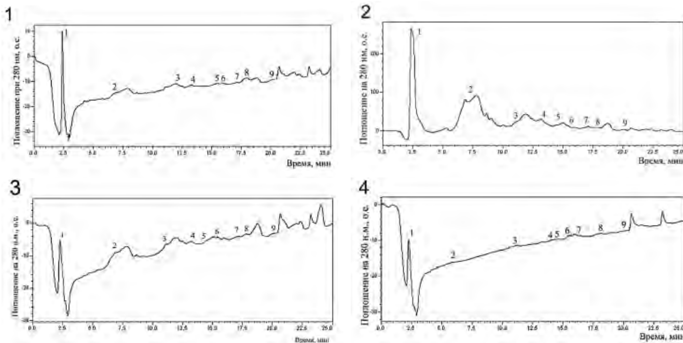
Рис. 5. Хроматограммы экспериментальных образцов жидких продуктов пиролиза: 1 – 350°C, нижняя фракция; 2 – 350°C, верхняя фракция; 3 – 400°C, нижняя фракция; 4 – 400°C, верхняя фракция
