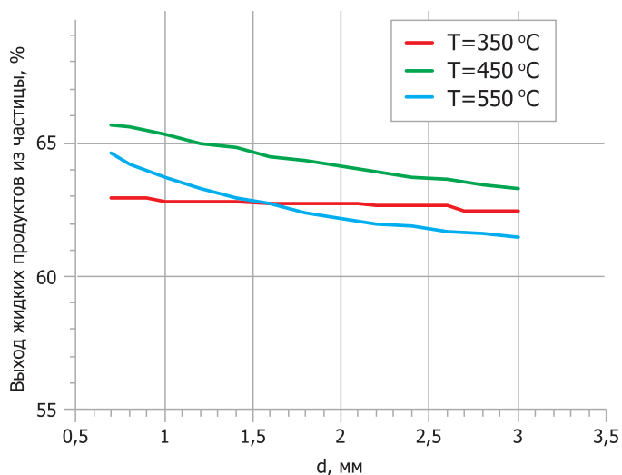
Рис. 2. Зависимость выхода жидких продуктов пиролиза из частицы биомассы влажностью 10% от радиуса частицы при различных температурах процесса
