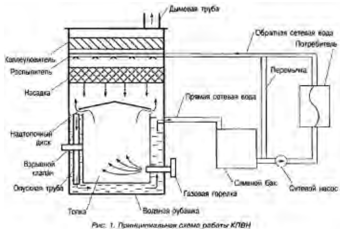
Рис. 1. Принципиальная схема работы КПВН
