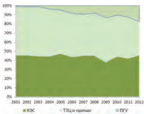
Рис 4. Динамика изменения коэффициентов использования установленной мощности турбин
